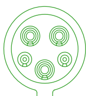
TYPE 1 SAE J1772-2009
